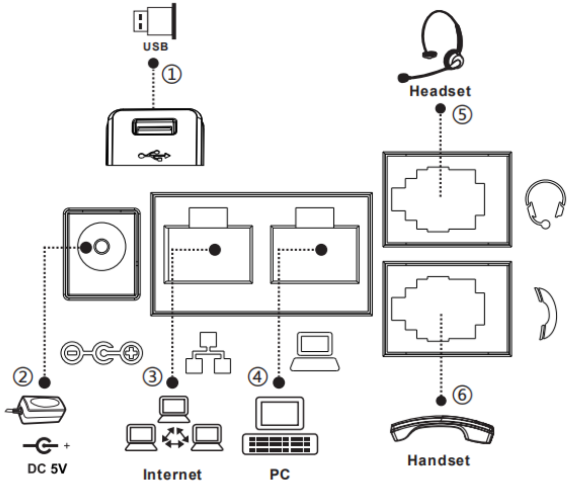
图 2 - 设备连接
